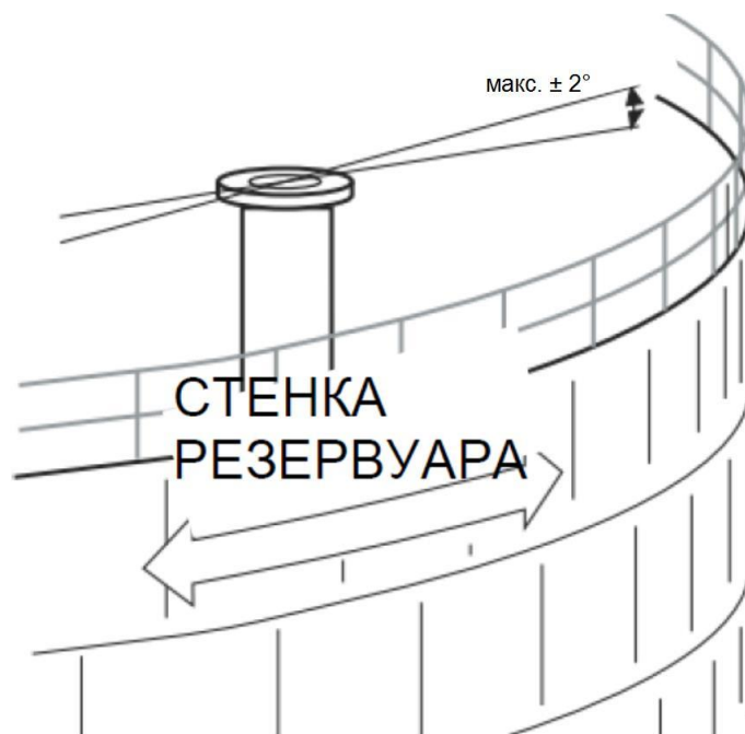
Рис.13 - Рекомендуемый вариант монтажа уровнемера на успокоительную трубу
