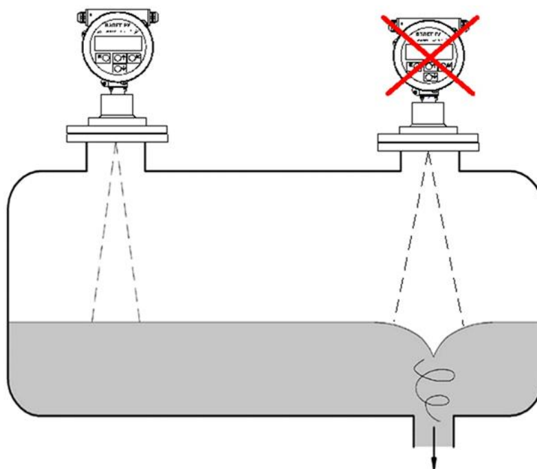
Рис.4 - Установка прибора на резервуар с выгрузкой продукта.
