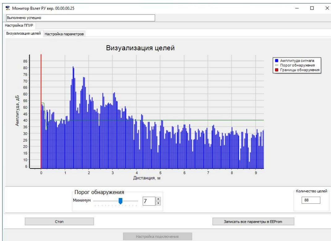
Рис.29 - Паразитные сигналы в шумовой дорожке.
