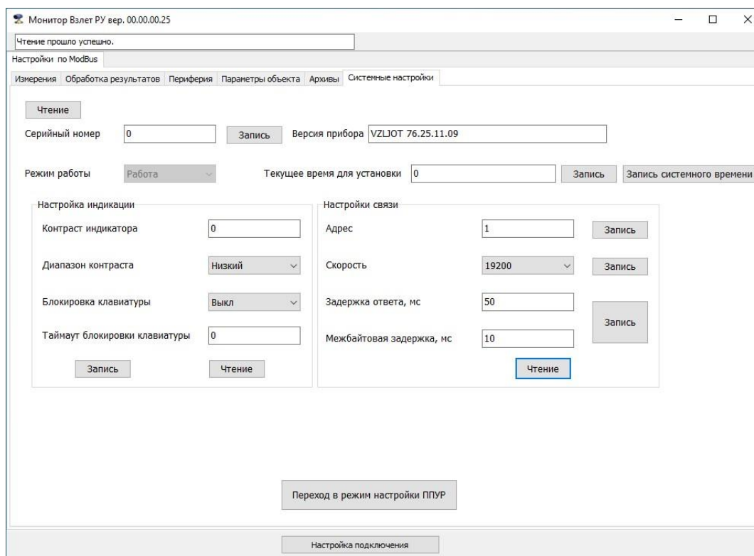
Рис.17 - Вкладка «Системные настройки».
