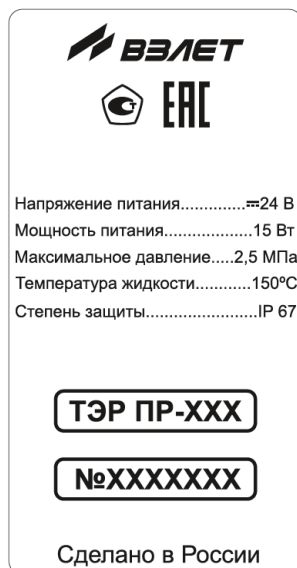
Рис.3. Вид шильда расходомера в едином конструктиве.
